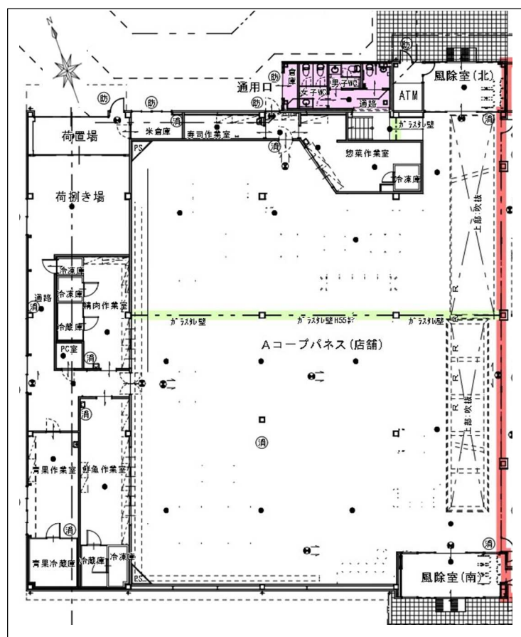
A コープパネス (1 階平面図)
